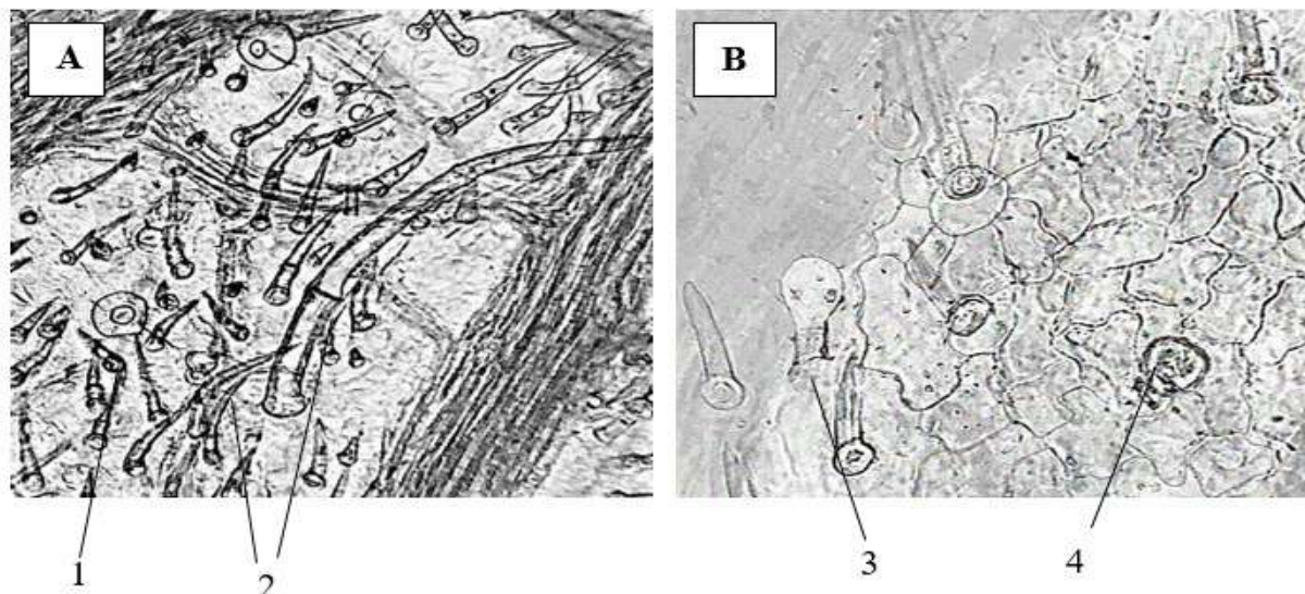
Рис. 4. Микроскопия чашелистиков L. deminutus (А, В – увеличение \times 100 ): А – поверхность зубца чашечки: 1 – эфиромасличная железка; 2 – простые многоклеточные волоски с бородавчатой кутикулой; В – нижний эпидермис чашечки: 3 – головчатый волосок с овальной головкой; 4 – головчатый волосок с округлой головкой
